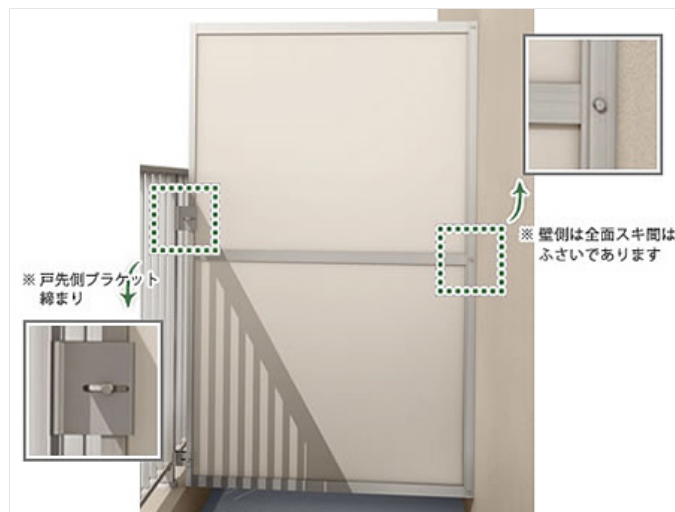
手摺取合
